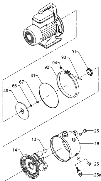
Obr. 6 Pohľad na rozložené čerpadlo
