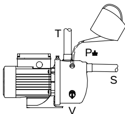
Fig. 5 Riempimento della pompa con acqua
