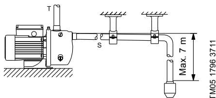
Slika 2 Cijevni priključci
