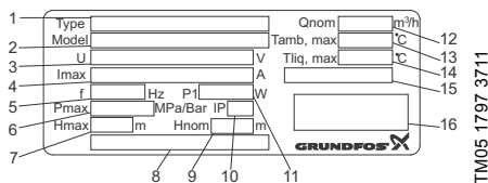
Fig. 1 Typskylt
