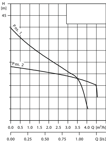
Рис. 3 Положіть кривої QH і клапану ежектора
