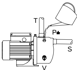
Fig. 5 Llenado de la bomba con agua
