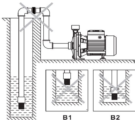
Schéma správné instalace B
