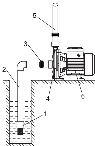
Schéma správné instalace A
